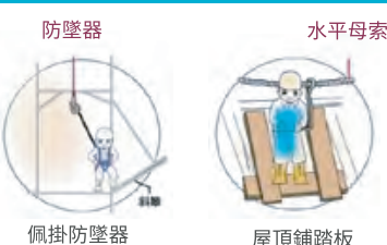
佩掛防墜器
