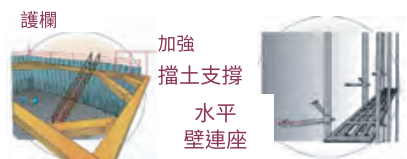
加強擋土支撐並設置護欄
